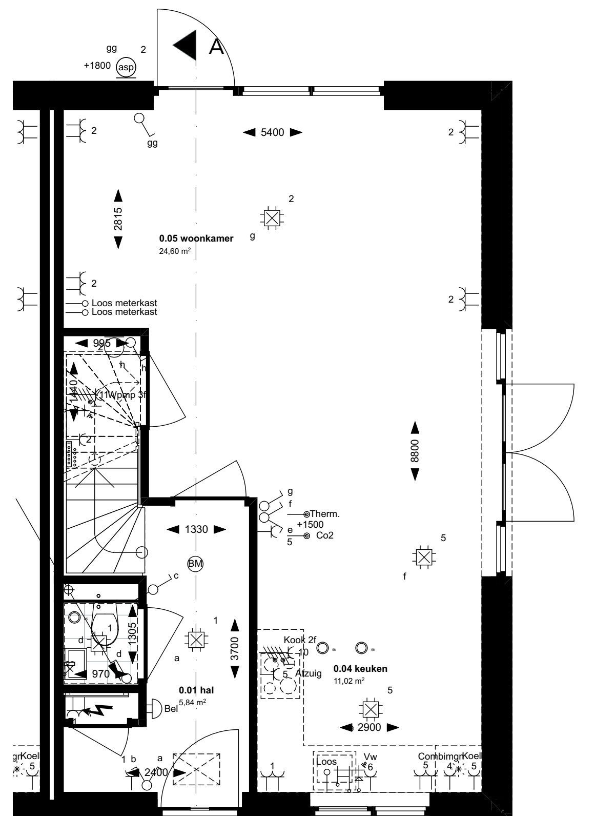
Begane grond
