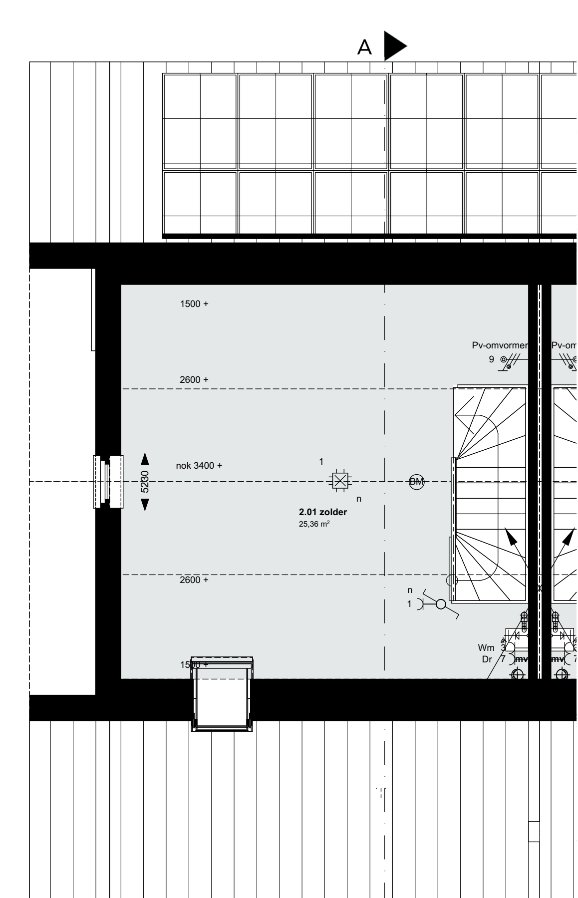
2e verdieping
