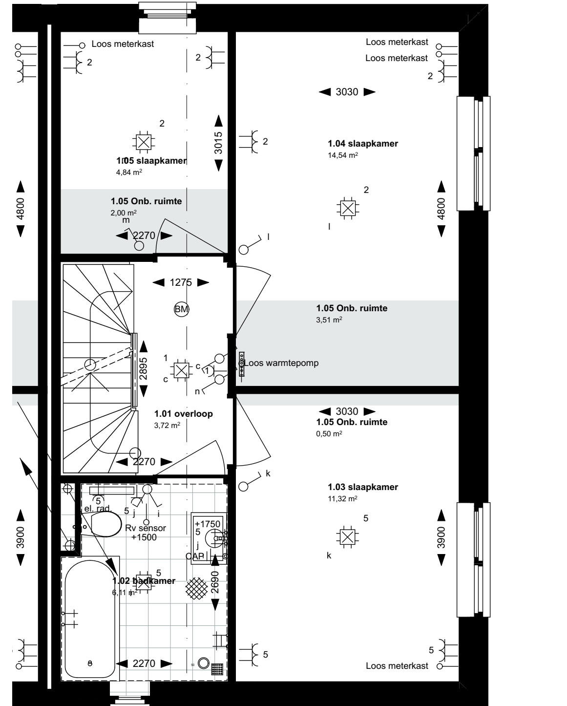
1e verdieping
