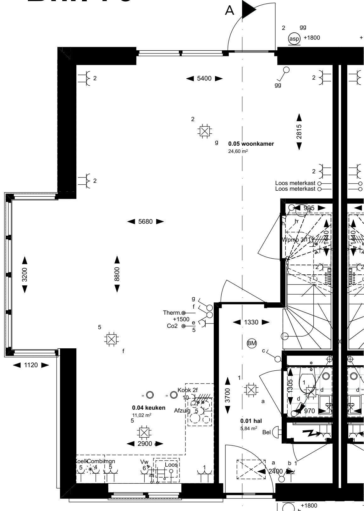
Begane grond
