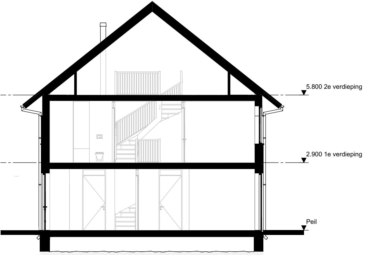
Doorsnede A
