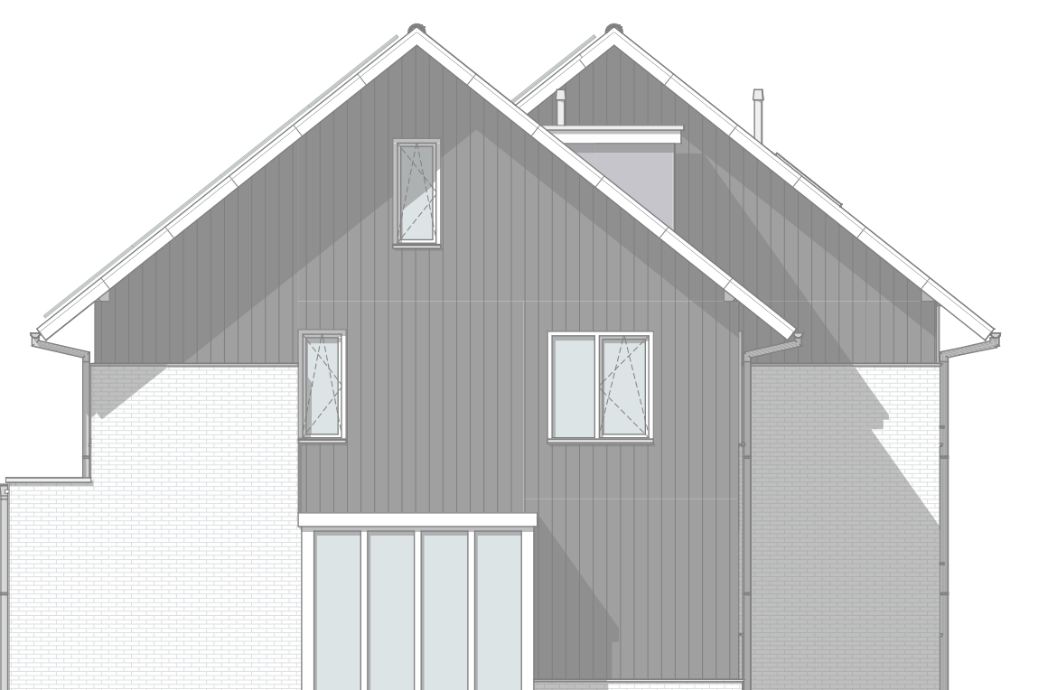
Linkergevel
