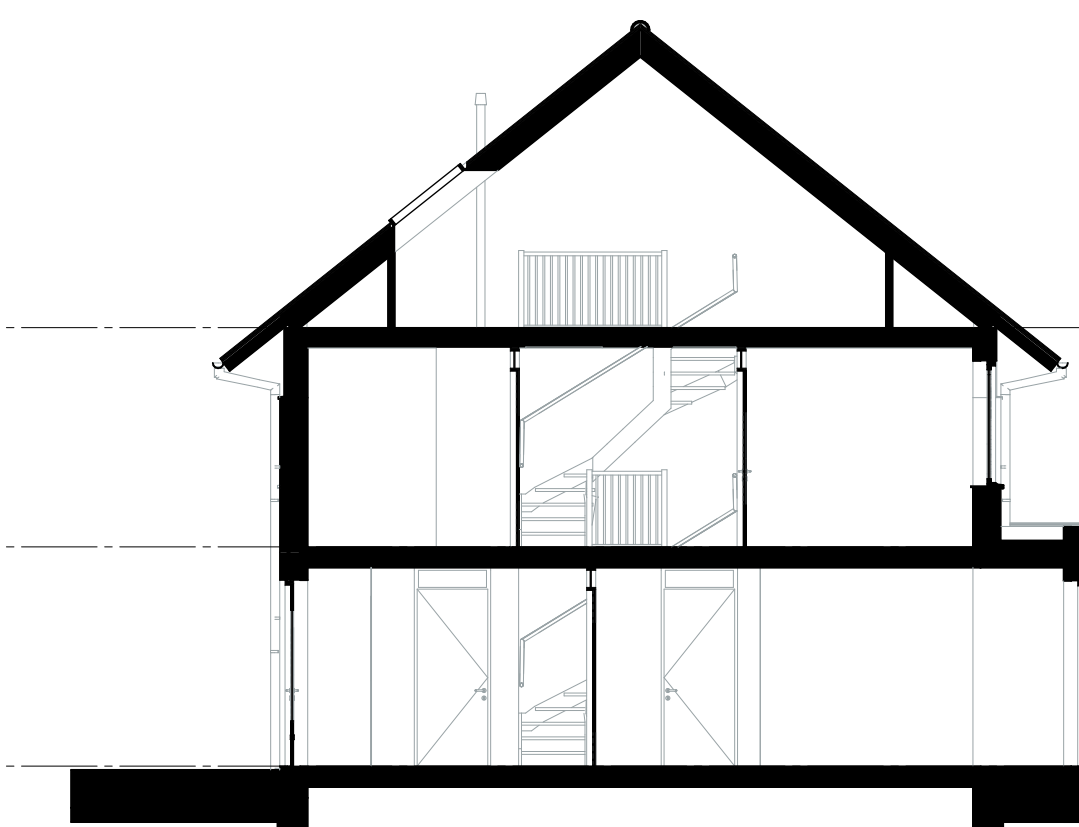
Doorsnede A
