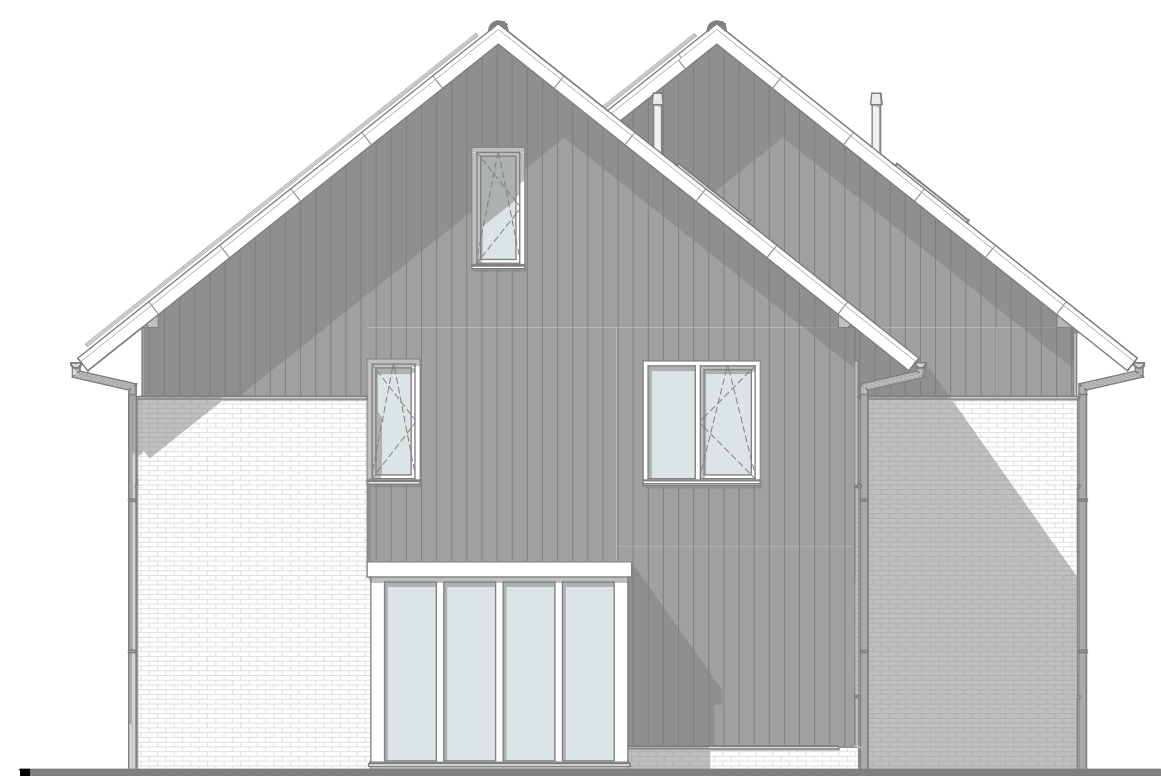
Linkergevel
