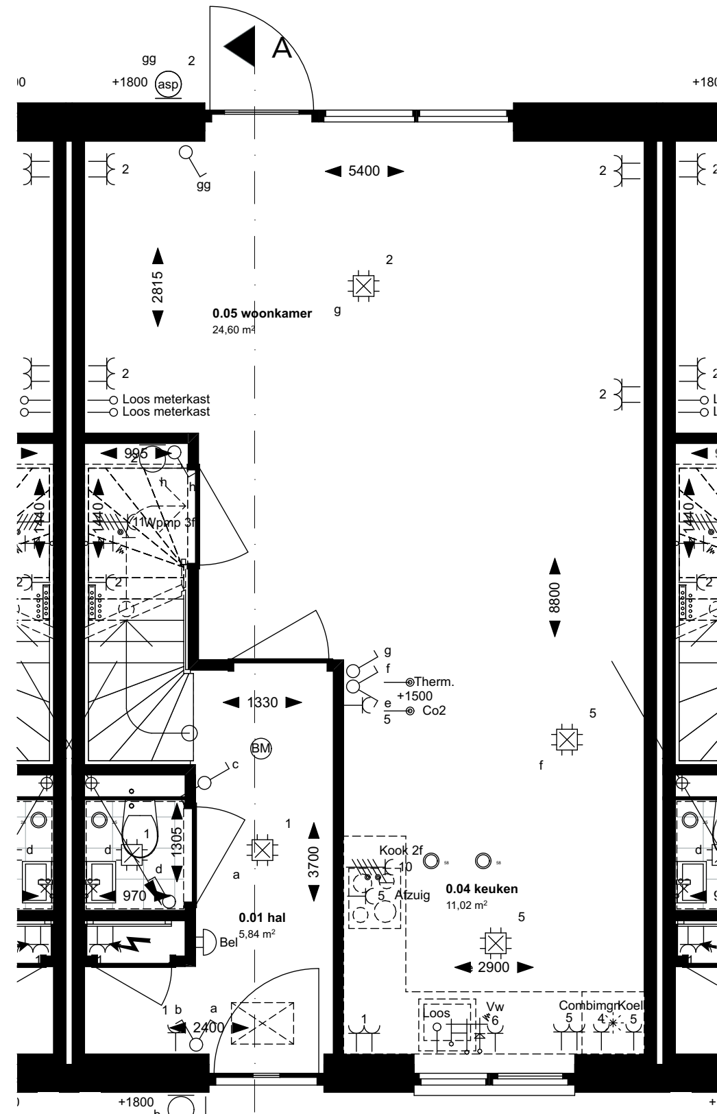
Begane grond
