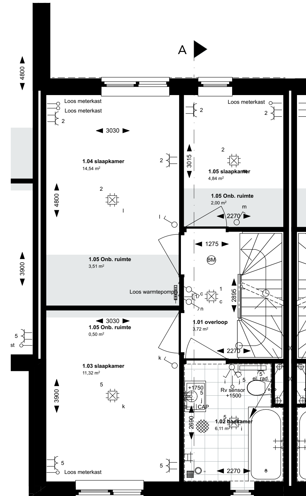
1e verdieping
