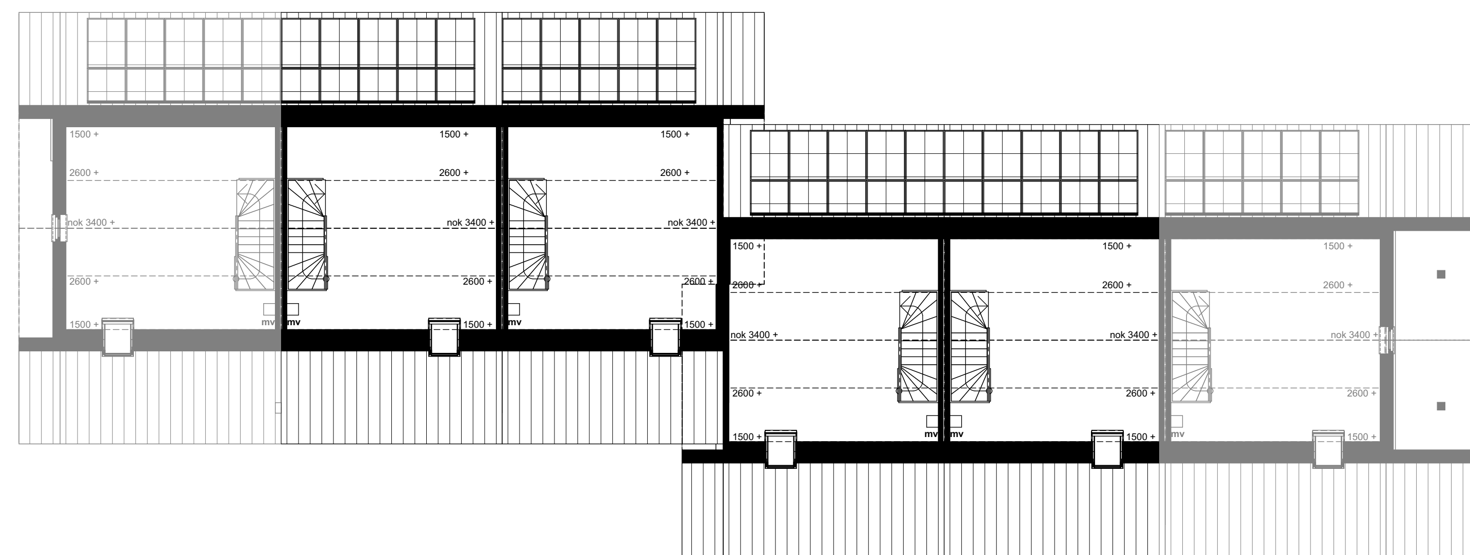
2e verdieping
