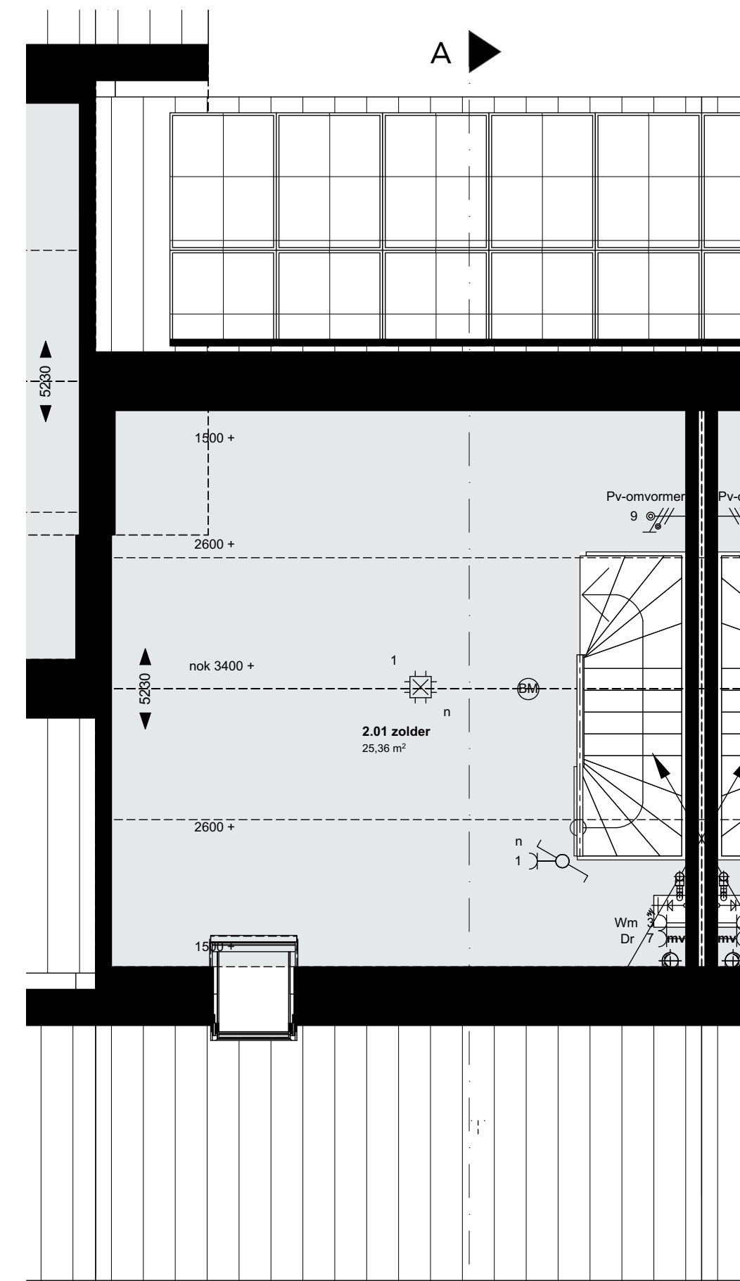
2e verdieping
