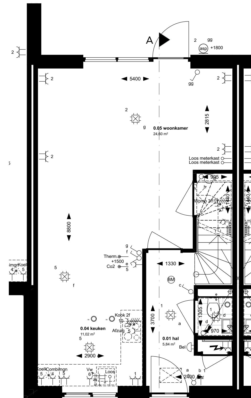
Begane grond
