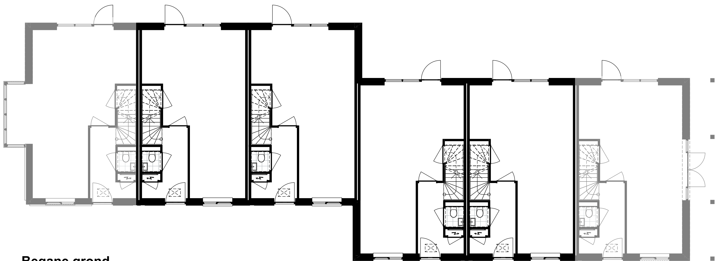
Begane grond
