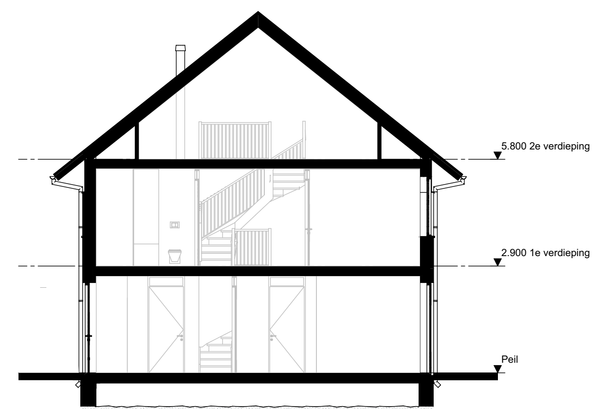
Doorsnede A
