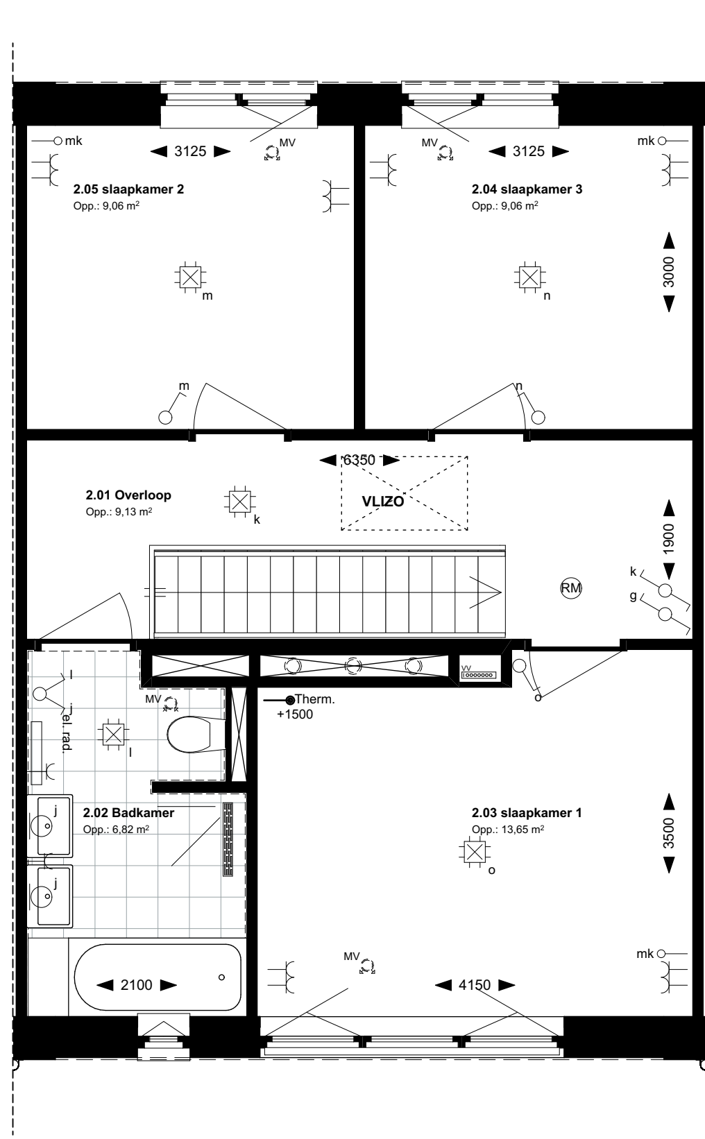
2e verdieping
