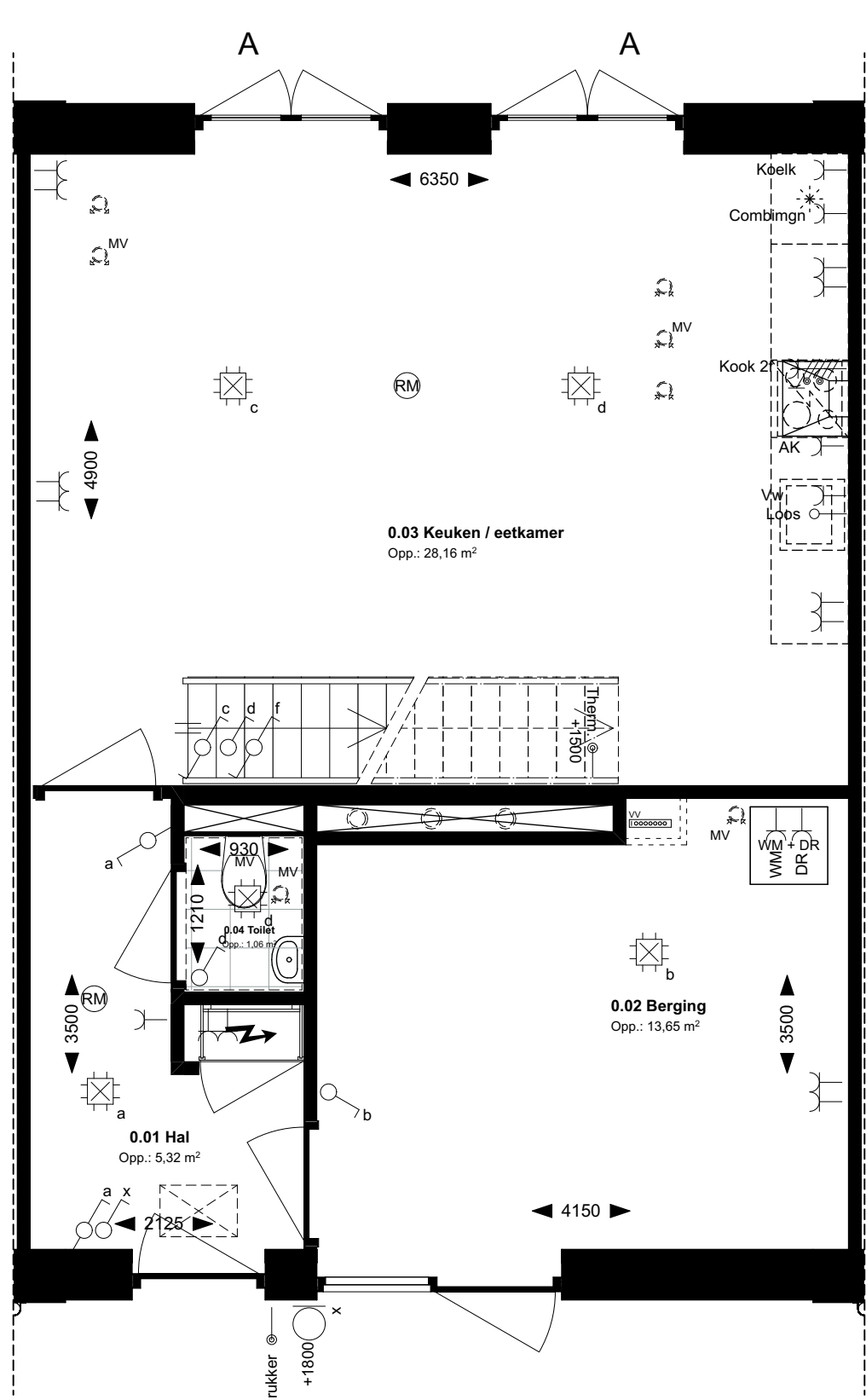
Begane grond
