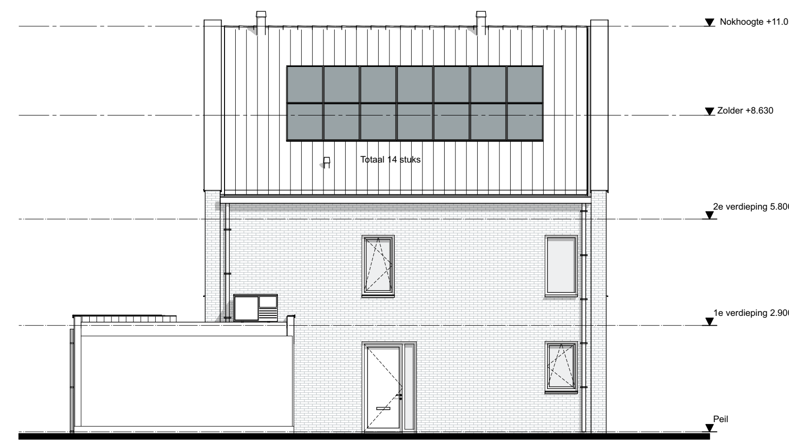
Linker zijgevel type C bnr 135, 137 & 139
