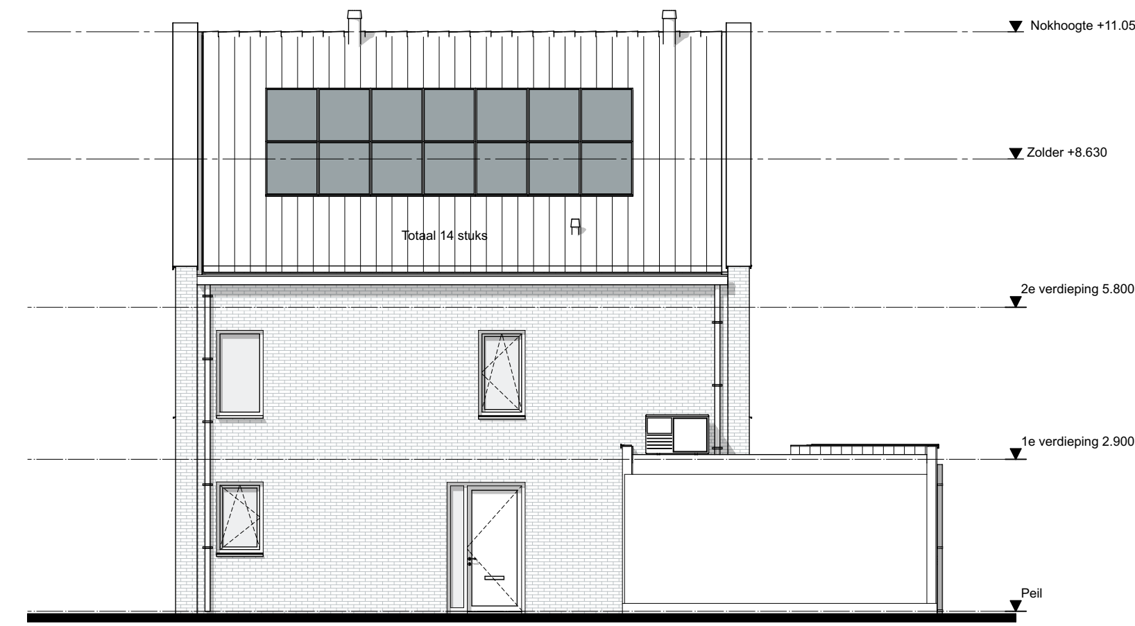
Rechter zijgevel type C 134, 136 & 138
