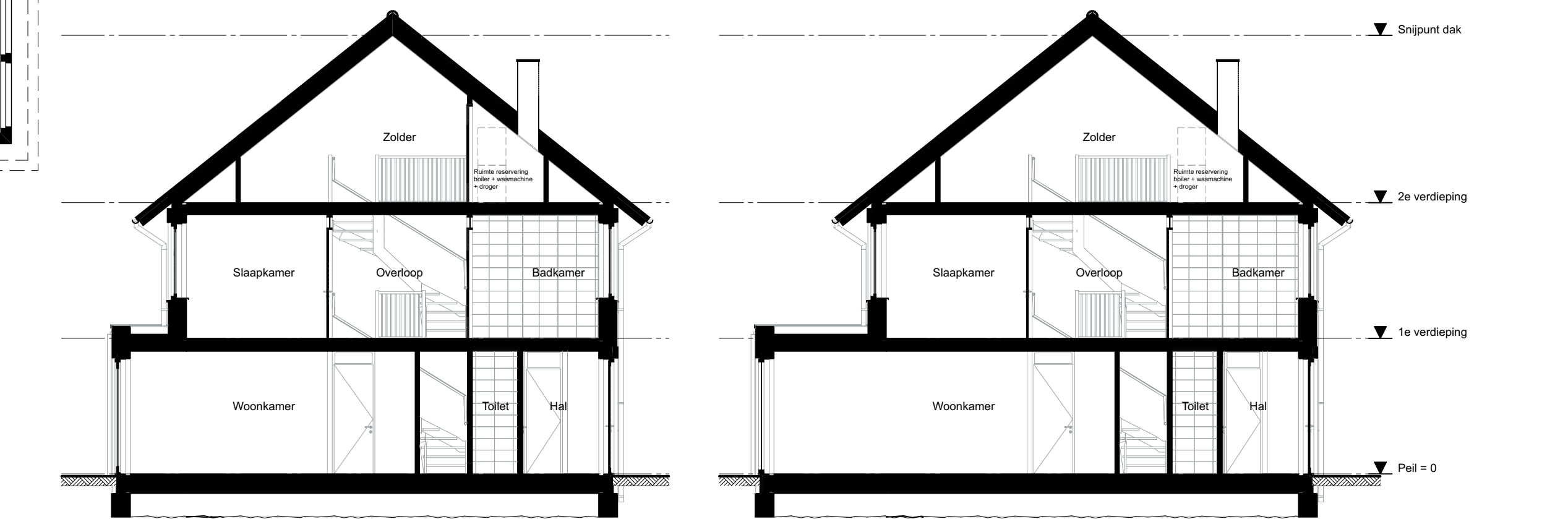
Doorsnede uitbouw 1,2m
