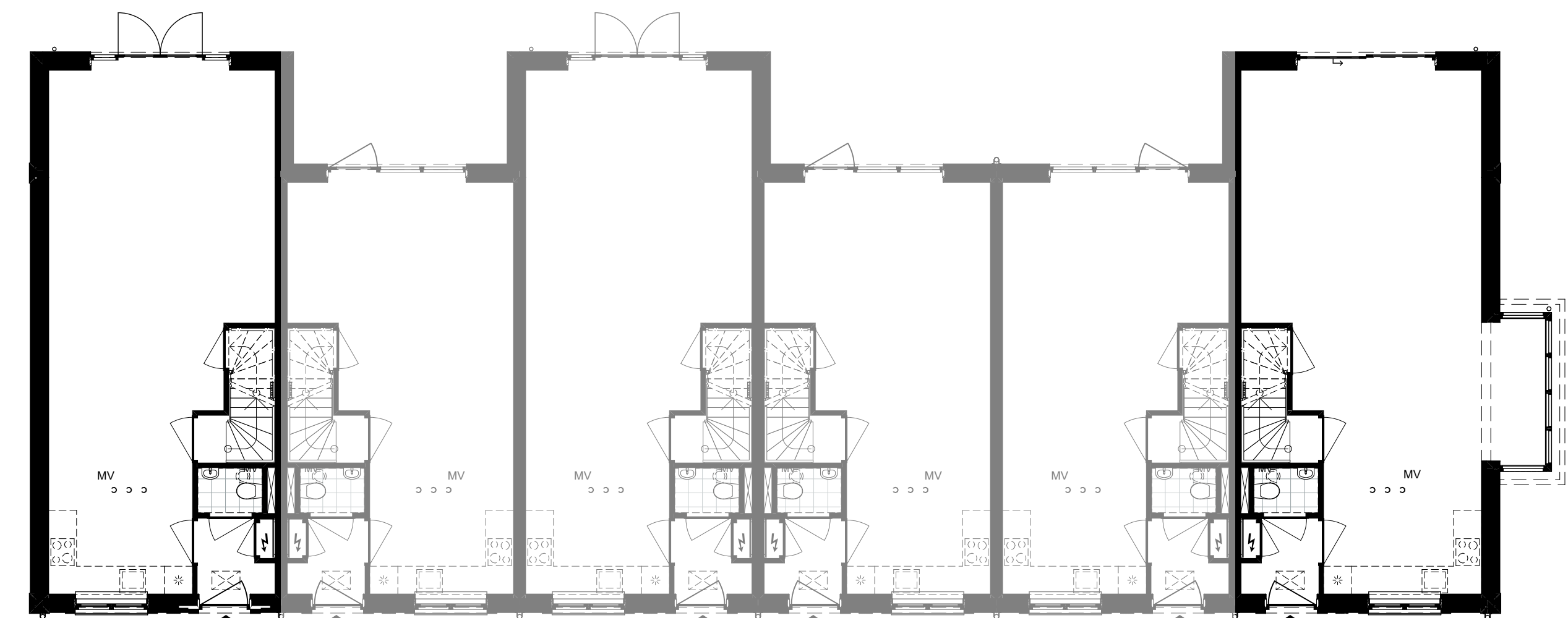
Begane grond opties
