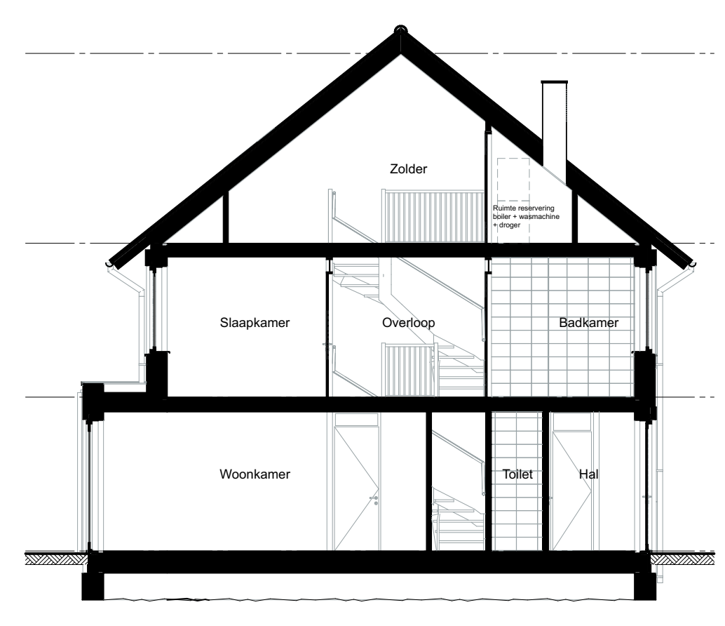
Doorsnede uitbouw 1,2m
