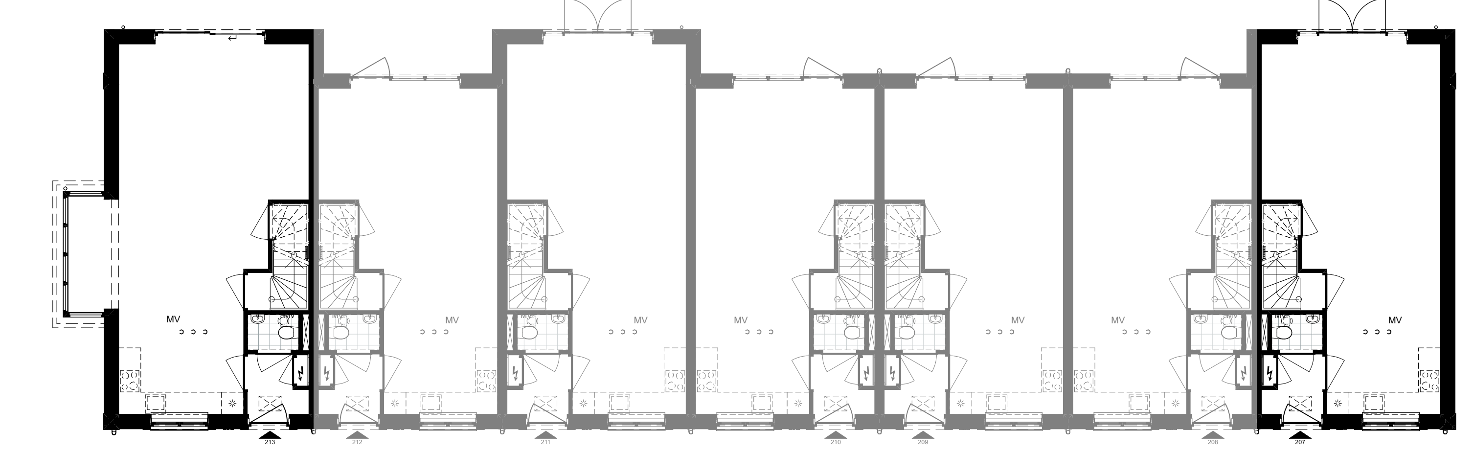
Begane grond opties
