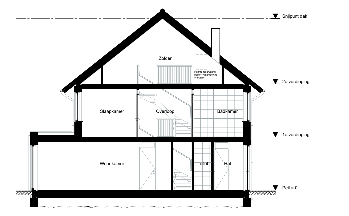
Doorsnede uitbouw 2,4m
